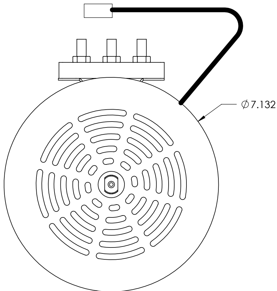
ENCODER END
