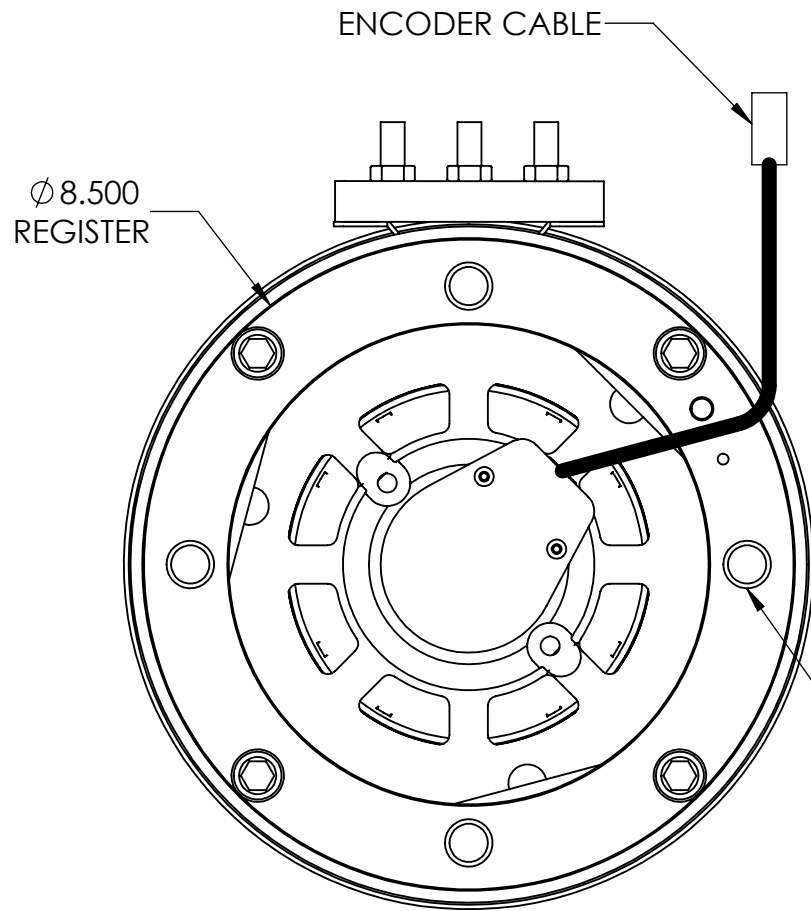
ENCODER END
