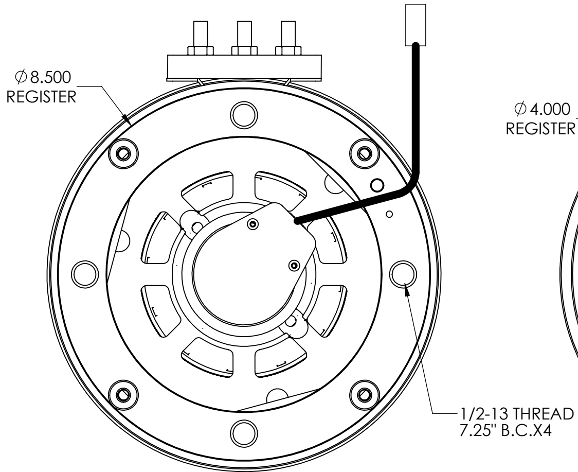
ENCODER END
