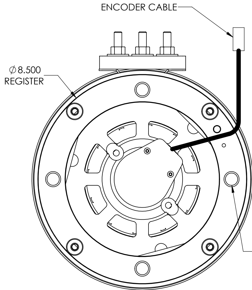
ENCODER END
