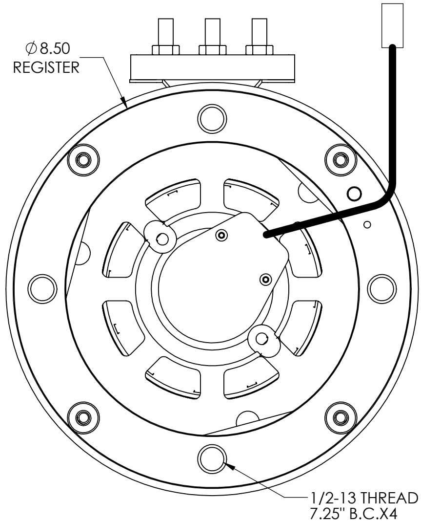
ENCODER END
