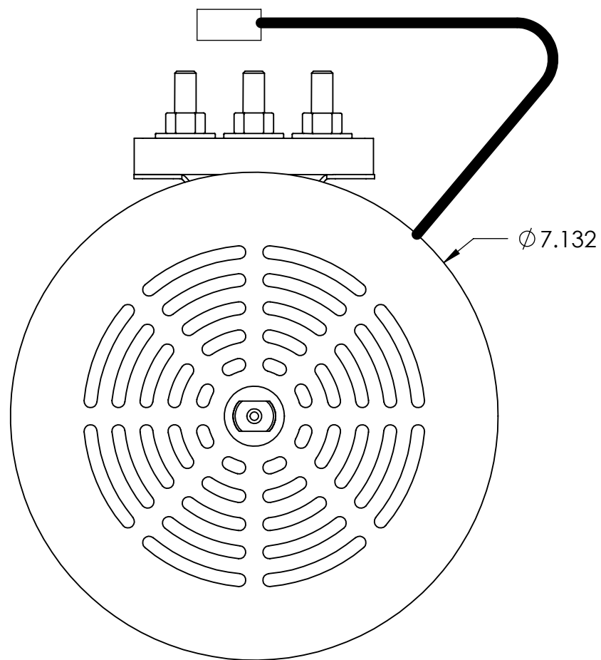
ENCODER END
