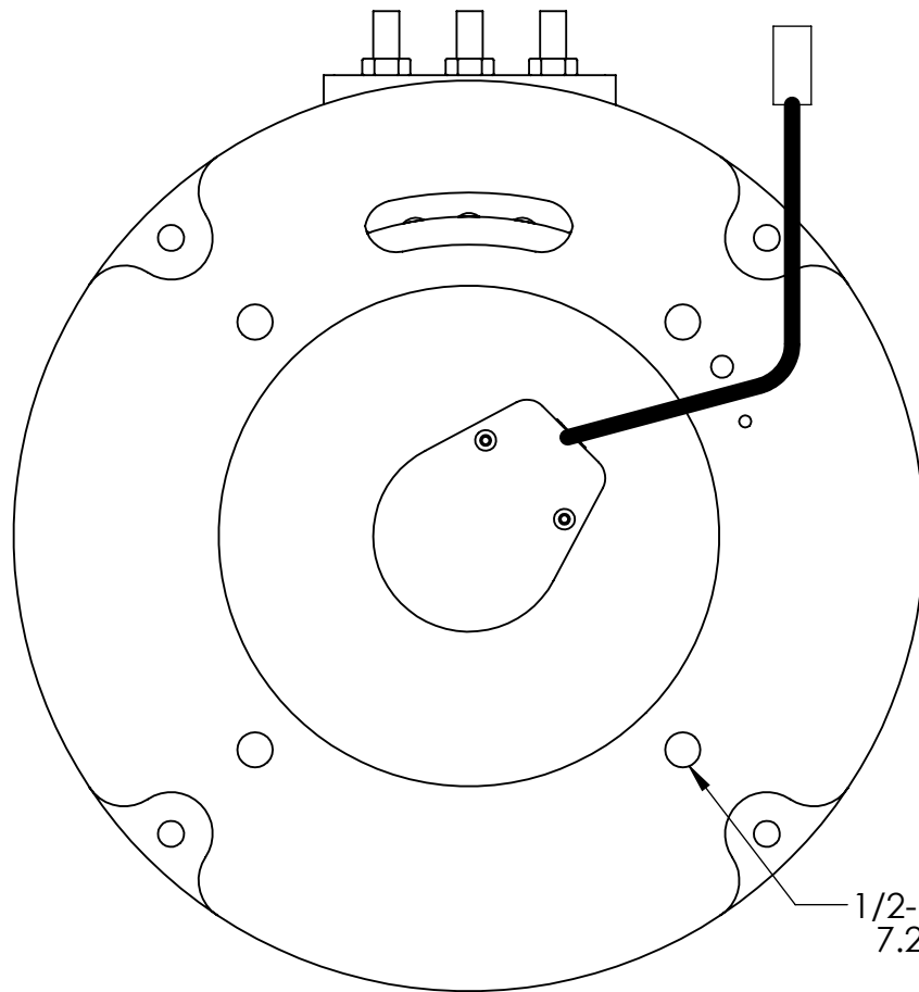
ENCODER END
